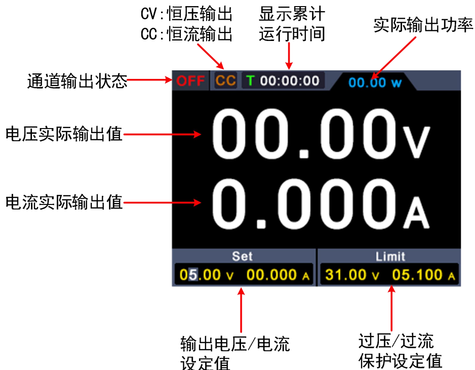
图 3-4 用户界面
