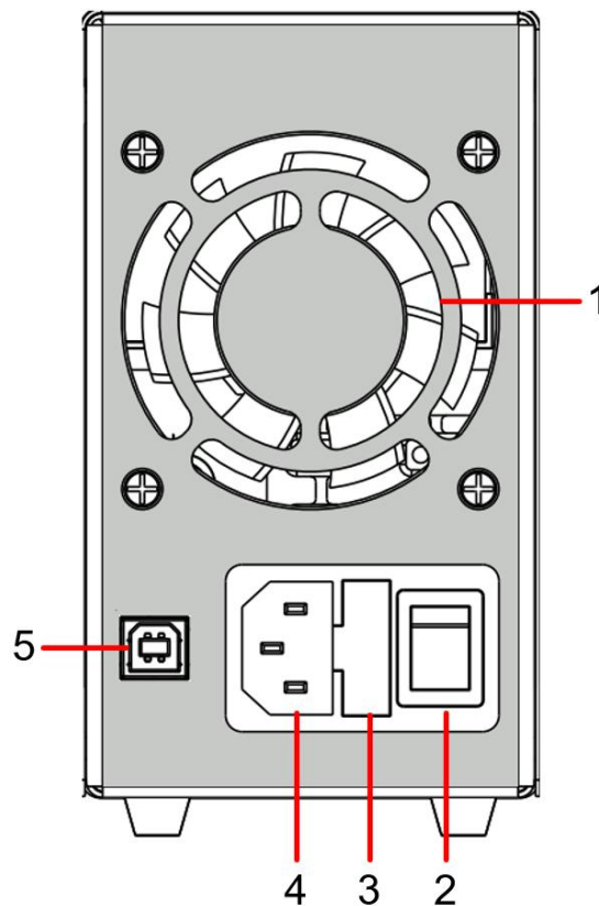
图 3-2 后面板概览
