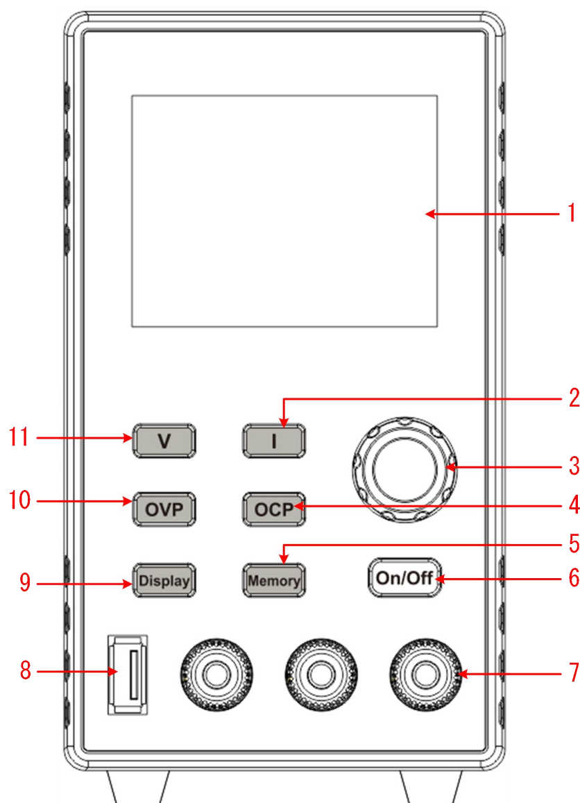
图 3-1 前面板概览
