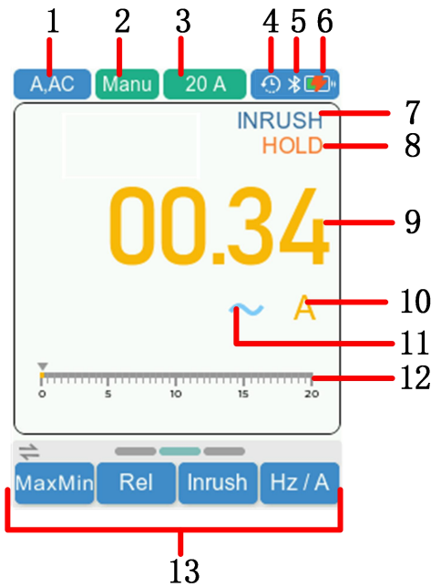
图 4-1：万用表界面
