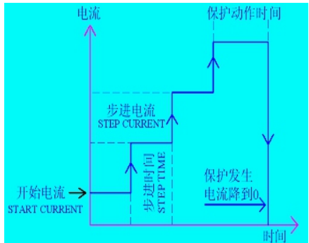
过流保护测试流程示意图
