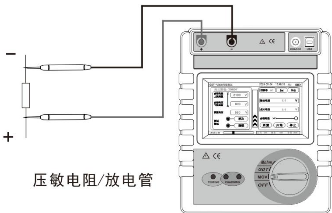
图 1（接线示意图）
