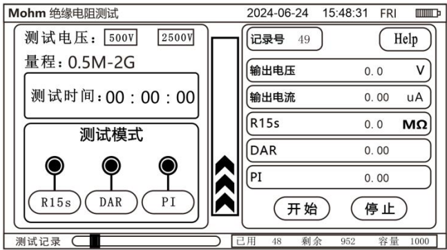
图 8（绝缘电阻测试界面）
